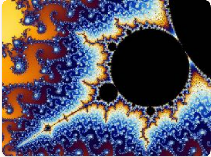
Ensemble de Mandelbrot
